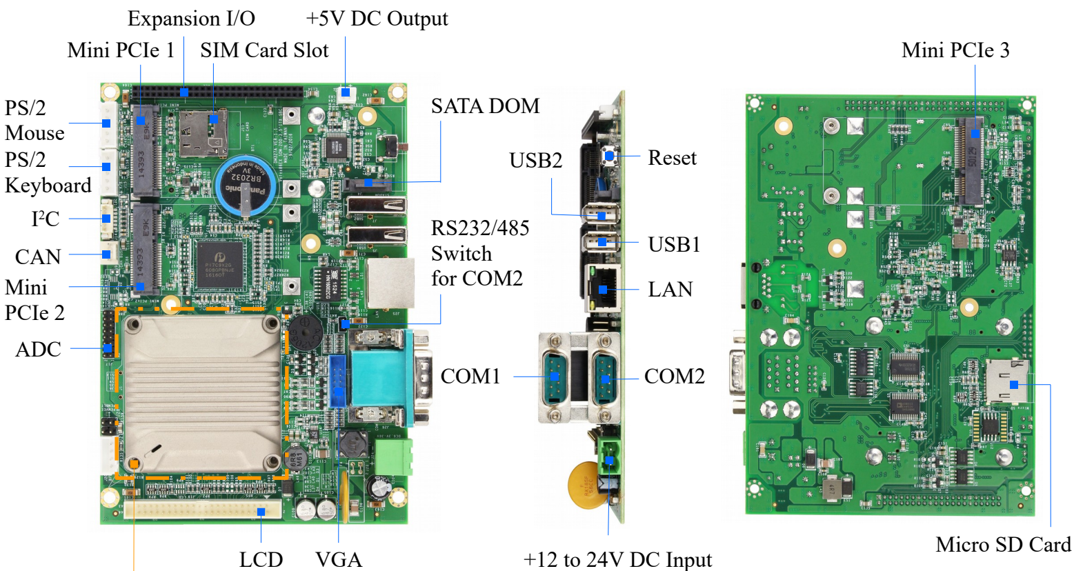
SOM200EX Module
